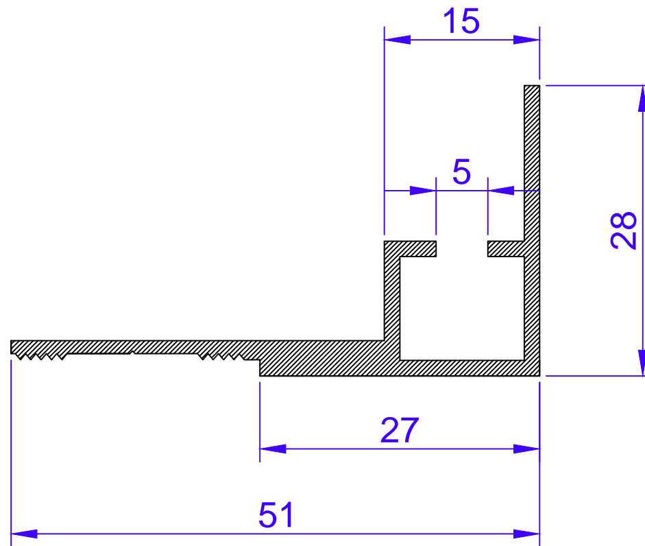
ALD-02 Right angled edge trim. Length 2.5m, 5m
